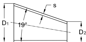
ekscentrični/eccentric/exzentrisch
